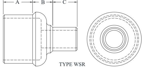
TYPE WSR
